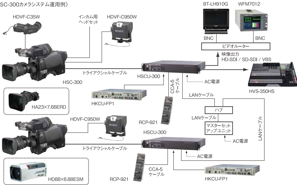
《HSC-300カメラシステム運用例》
